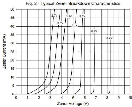
Zener current vs Zener voltage
