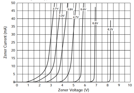
Zener current vs Zener voltage
