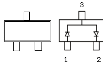
SOT-23
