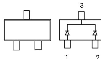
SOT-23
