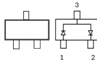
SOT-23
