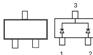
SOT-23
