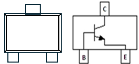
SOT-723
