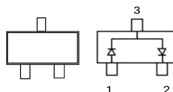
SOT-23
