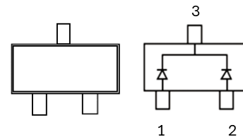
SOT-23
