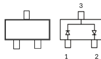
SOT-23
