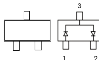
SOT-23
