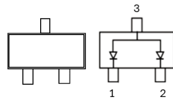
SOT-23
