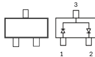
SOT-23
