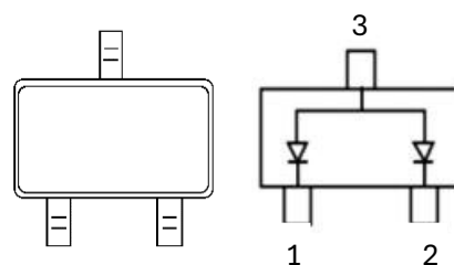
SOT-323
