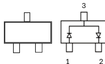
SOT-23
