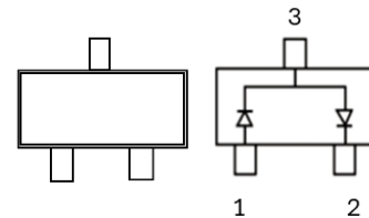
SOT-23
