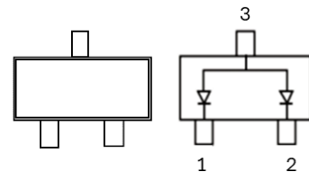
SOT-23
